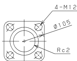
吐出しフランジ
