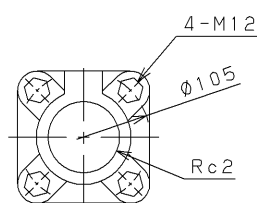
吸込フランジ
