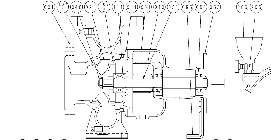
グランドパッキン仕様 (特殊仕様) GLAND PACKINGS SPECIFICATION (OPTION)
